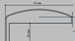
Наличник полукруглый телескопический
