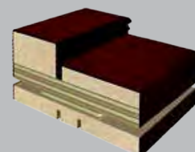
Коробка прямая телескопическая
