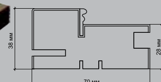
Коробка прямая заподлицо телескопическая
